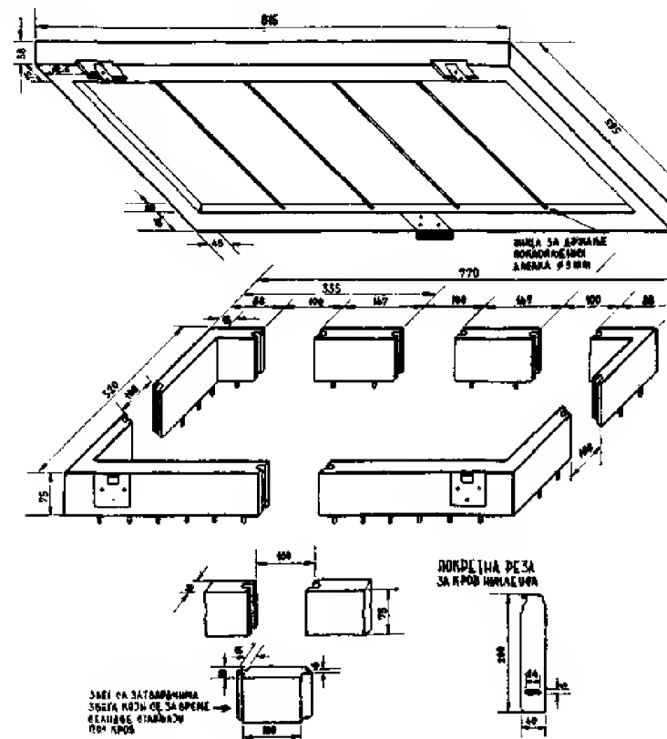
Начин израде збег и крова за нуклеус
